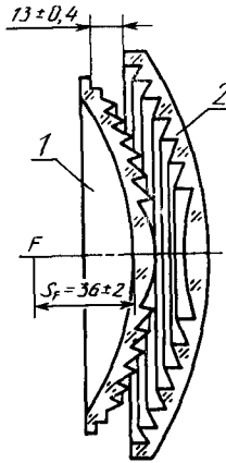
1 — светофильтр-линза СЛ-139 М; 2 — линза ступенчатая ЛС 160
