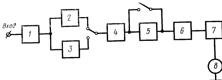
Схема преобразования измерительного сигнала детонетром
