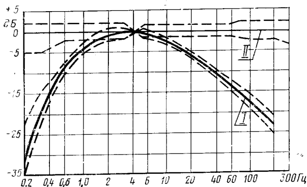
Частотные характеристики детонатора
