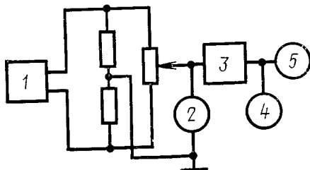
Схема проверки вспомогательного устройства
