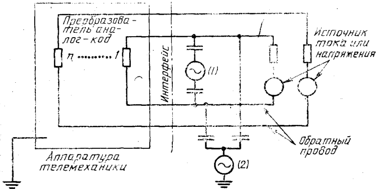
Схема для аналоговых входных сигналов
