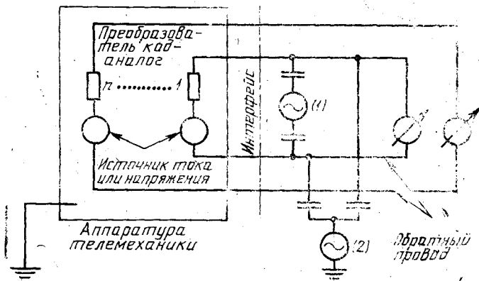
Схема для аналоговых выходных сигналов
